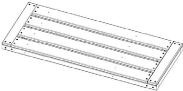
TP03 ASSEMBLAGE DE TABLE MOYENNE COURTE - W2A03995 (x1) 2 1/16 po x 16" x 39 1/2 po (52x407x884)
