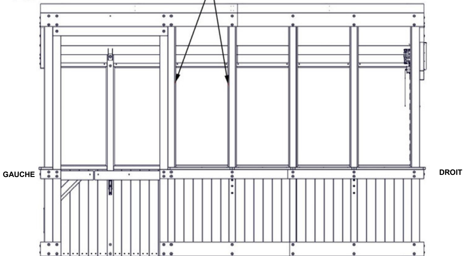
681 (x8) CANAL EN POLY AVEC RUBAN
