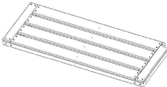
TP04 ASSEMBLAGE DE TABLE GAUCHE - W2A03996 (x1) 2 1/16 po x 16 po x 41 1/2 po (52x407x934)
