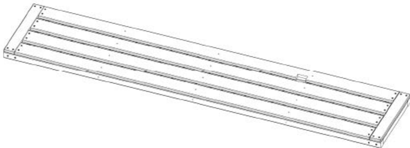
TP01 ASSEMBLAGE DE TABLE DROITE - W2A03993 (x1) 2 1/16 po x 16 po x 80 7/16 po (52x407x1923)
