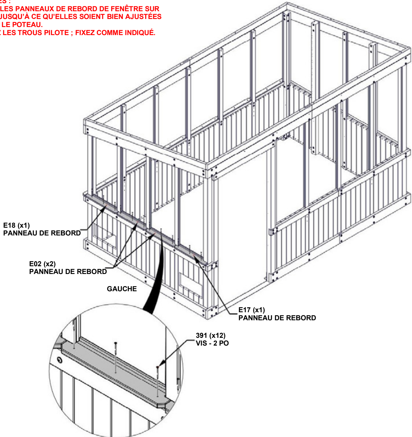
E02 PANNEAU DE REBORD - W4L18694 (x2) 1 7/16 po x 3 3/8 po x 19 15/16 po (36x86x507)
