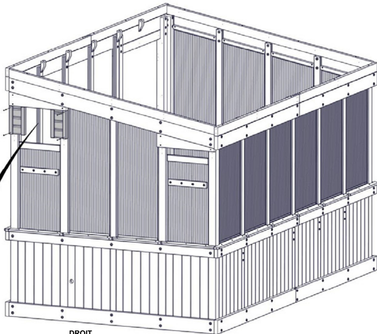
FT01 (x1) ASSEMBLAGE DE GARNITURE DE VENTILATEUR - W2A03987 17/16 PO X 65/16 PO X 10 9/16 PO (36x160x268)
