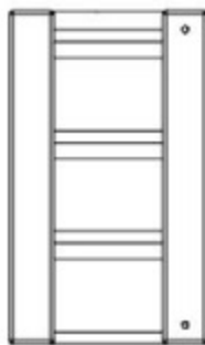
FT02 (x1) ASSEMBLAGE DE GARNITURE DE VENTILATEUR - W2A03988 17/16 PO X 65/16 PO X 10 9/16 PO (36x160x268)
