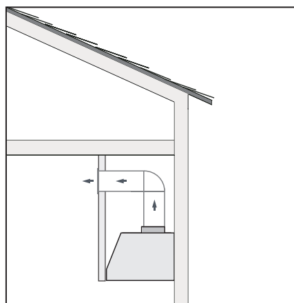
ÉVENT D'ÉCHAPPEMENT DE SOFFITE
