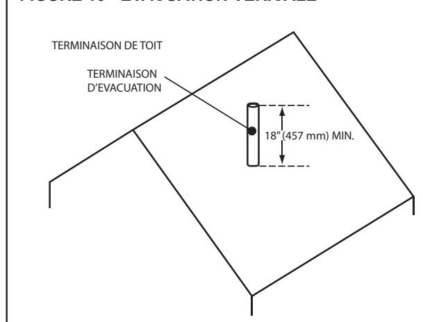
FIGURE 10 - ÉVACUATION VÉRICALE
