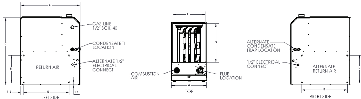
FIGURE 1 - DIMENSIONS DE LA FOURNAISE ET DÉGAGEMENTS AUX MATÉRIAUX COMBUSTIBLES
