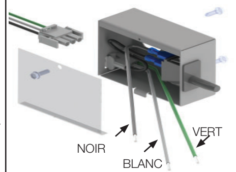
FIGURE 28 - BRANCHEMENT ÉLECTRIQUES / CONNECTEUR MOLEX
