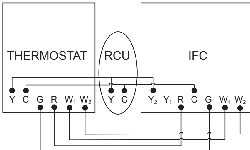
FIGURE 31 - DIAGRAMME DU CONNECTEUR DU THERMOSTAT
