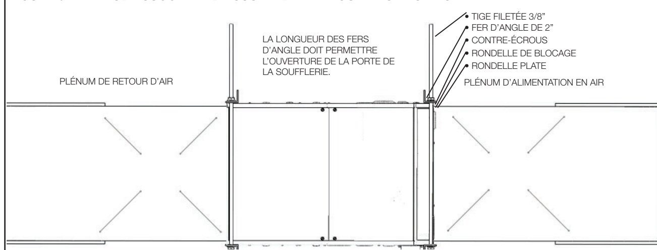
FIGURE 3 - MÉTHODE SUGGÉRÉE DE SUSPENDRE LA FOURNAISE HORIZONTALE
