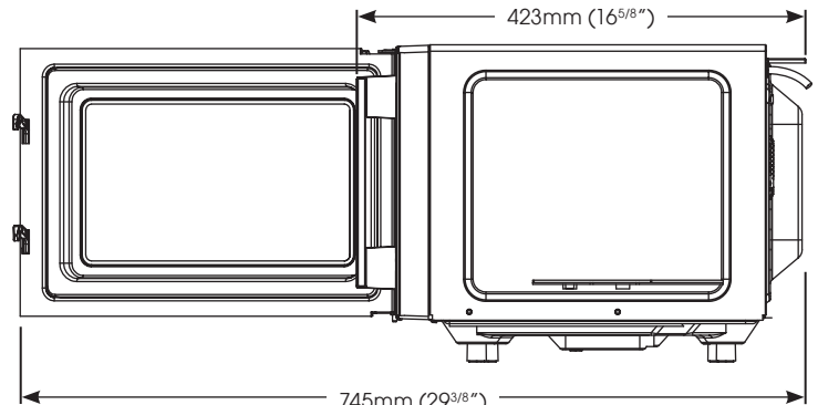
VISTA LATERAL CON LA PUERTA ABIERTA
