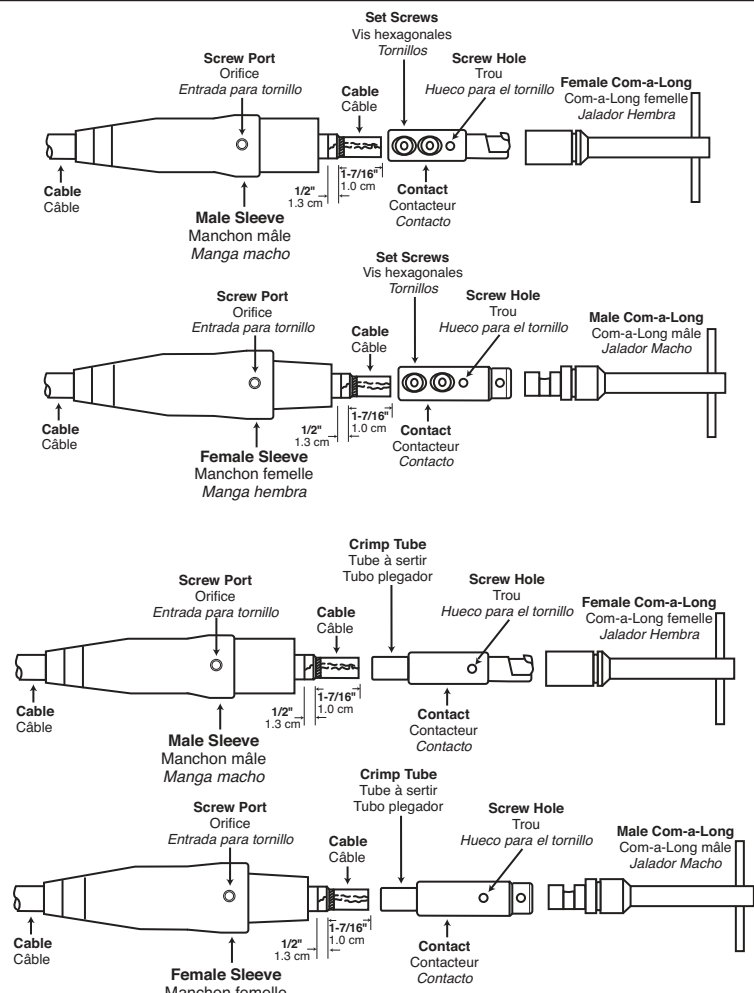
Figure 1 / Figura 1 16 Series Male and Female - Set Screw Connecteurs mâles et femelles à visser (série 16) Macho y Hembra Serie 16 - Tornillo
