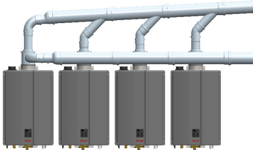
Figura 47: Ejemplo: Ventilación común Rinnai
