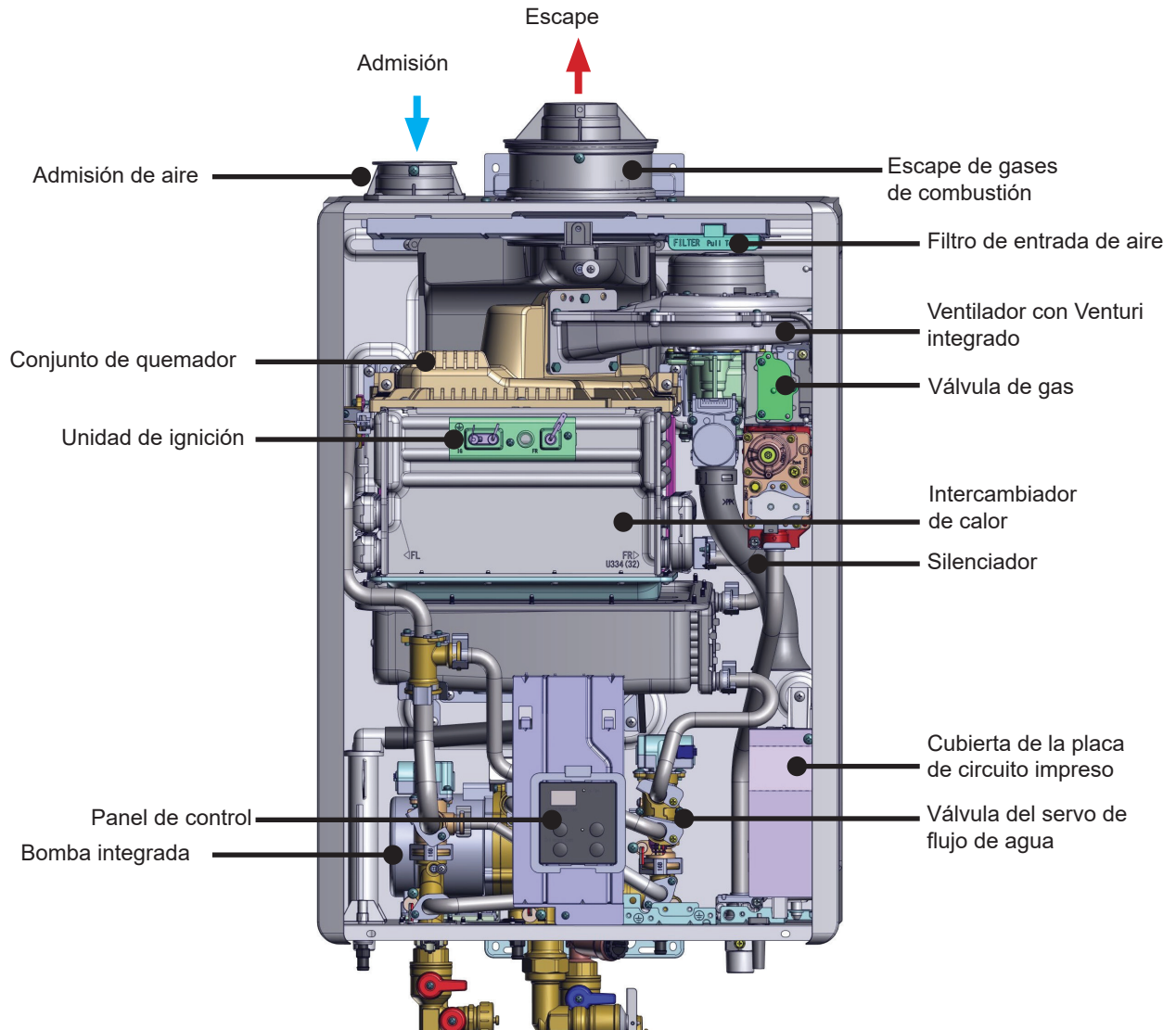
Figura 3: Componentes
