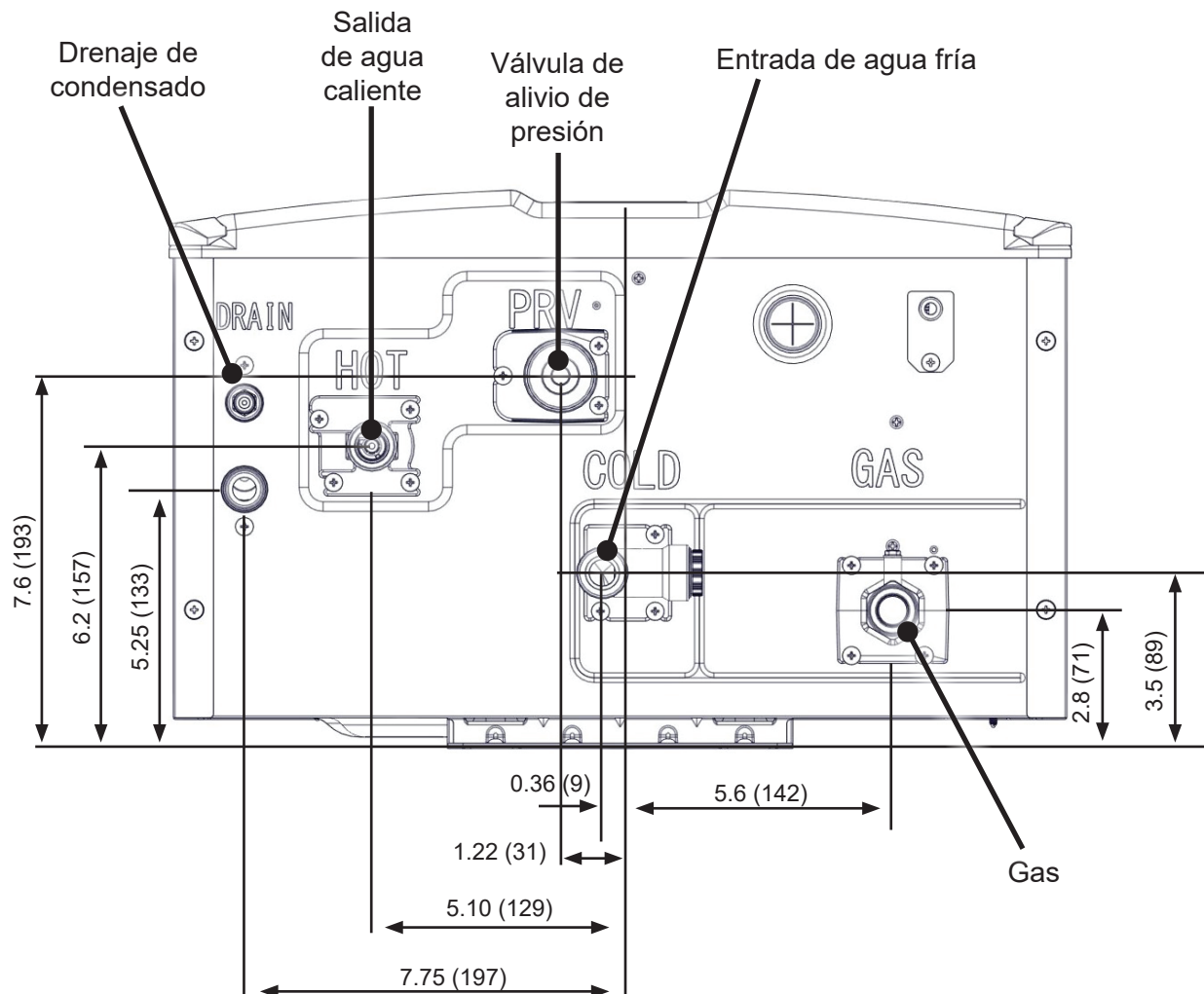
Figura 6: Conexiones de suministro
