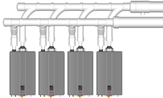
Figura 48: Ejemplo: Ventilación común de PVC/CPVC Schedule 40
