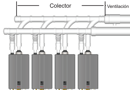
Figura 50: Instalación de ventilación común de PVC/CPVC
