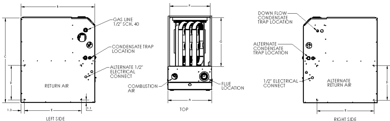
TABEAU A - DIMENSIONS DE LA FOURNAISE
