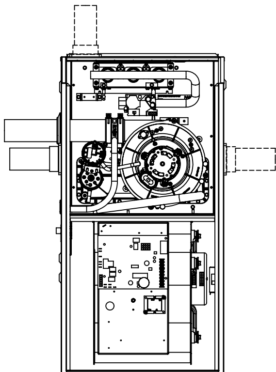
ÉVENT GAUCHE - ÉVACUATION GAUCHE INSTALLATION (INTERNE)
