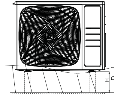
Installation incorrecte
