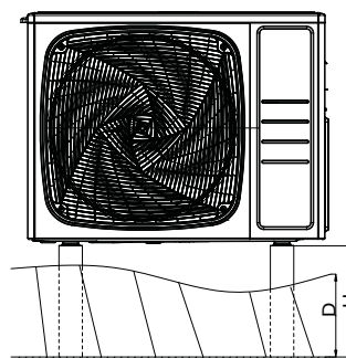
Instalación correcta
