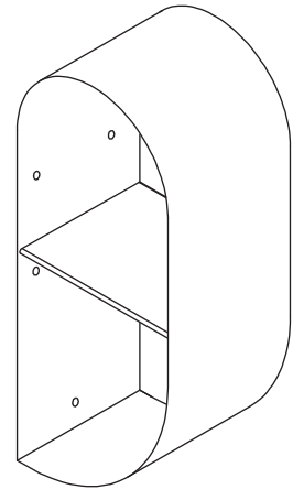
RIGHT SHELF ESTANTE DERECHO ÉTAGÈRE DROIT
