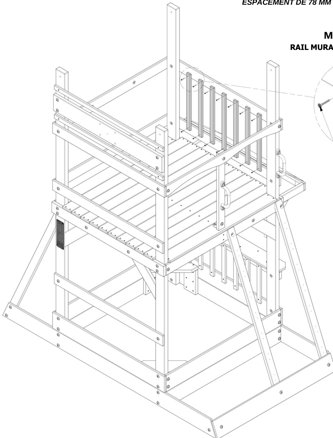
088 (x14) VIS - 1 1/8 "
