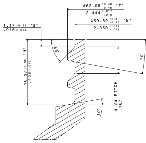
Section cut B-B Scale: 8:1
