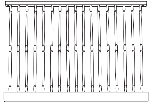
C. Crib Side (2) C. Côté du lit de bébé (2)
