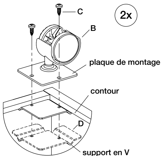
FIGURE 4 : Vue rapprochée du montage de roulette arrière.
