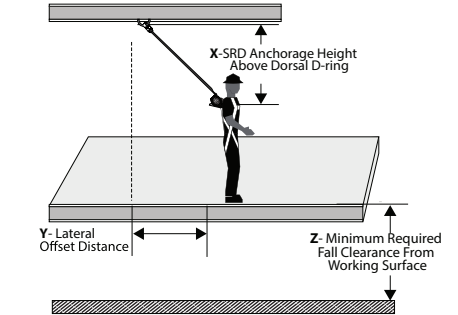
Figura 15 - Distancia despejada de caída mínima requerida de FT-X para usuarios de 310 a 420 libras (141 a 191 kg)
