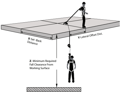
Figure 14 - Ancrage non aérien pour le dégagement minimal requis en cas de chute (DMC)
