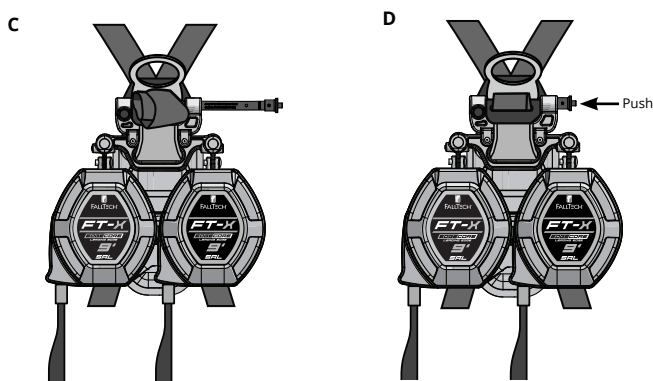
Figure 6 - Installation du bord d'attaque SRL-P de classe 2 FT-X EdgeCore avec applications d'arrimage à arc électrique
