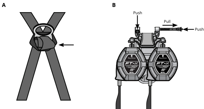
Figure 6 - Installation du bord d'attaque SRL-P de classe 2 FT-X EdgeCore avec applications d'arrimage à arc électrique
