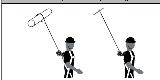
Figure 3 - Connexions d'ancrage acceptables pour le dispositif avec bord d'attaque à arc électrique FT-X EdgeCore
