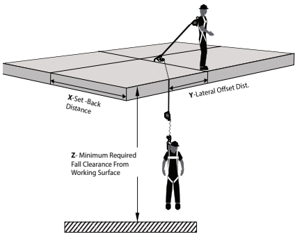
Figura 12 - Distancia despejada de caída mínima requerida de FT-X para usuarios de 130 a 310 libras (59 a 141 kg)
