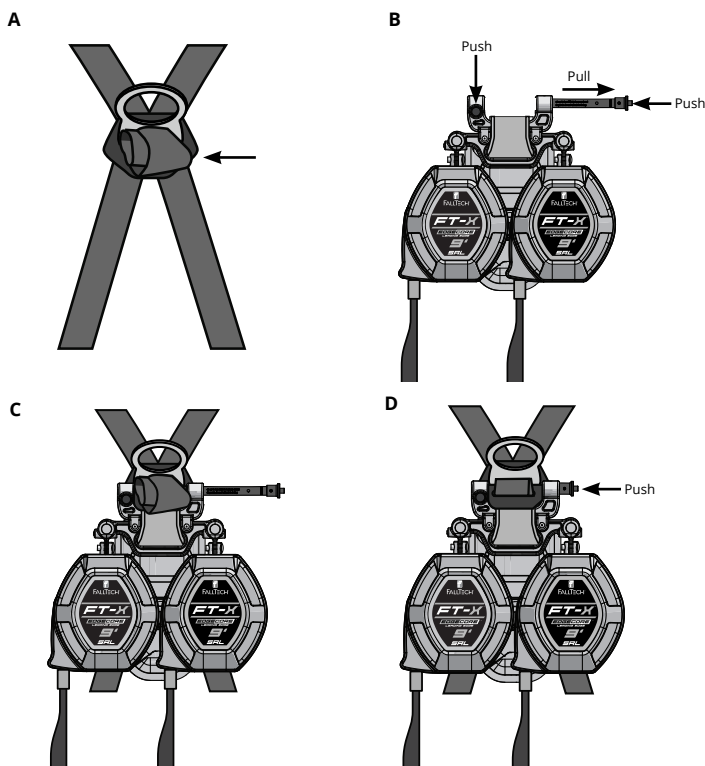
Figura 6 - Instalación de FT-X EdgeCore de Amarre Arco Eléctrico Class 2 Leading Edge SRL-P
