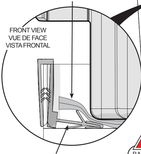
Gasket on the bathtub side flange Joint sur la bride de côté de la baignoire Junta sobre la brida lateral de la bañera
