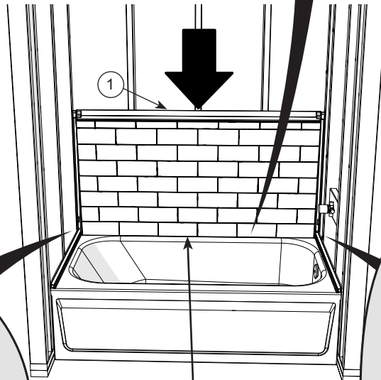
Gasket on the bathtub back flange Joint sur la bride arrière de la baignoire Junta sobre la brida trasera de la bañera
