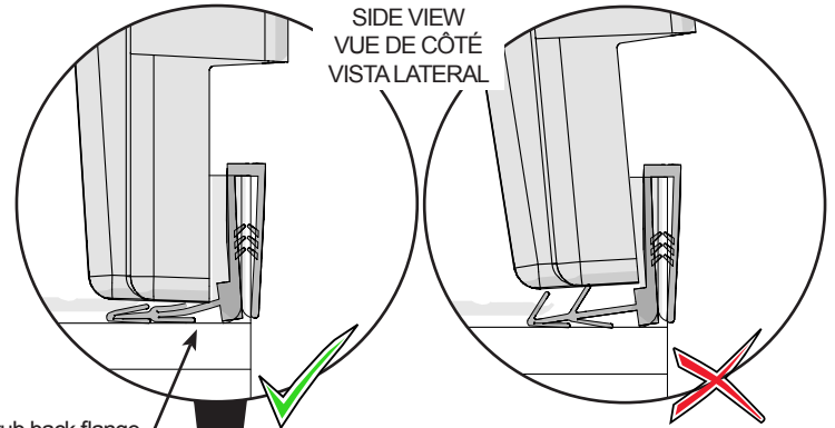
Gasket on the bathtub back flange Joint sur la bride arrière de la baignoire Junta sobre la brida trasera de la bañera
