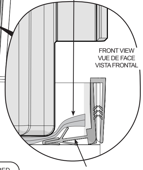
Gasket on the bathtub side flange Joint sur la bride de côté de la baignoire Junta sobre la brida lateral de la bañera
