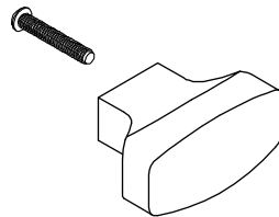
HANDLE M4 X 25 mm QTY 4 SETS
