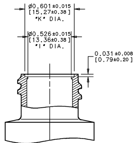
NECK DETAIL SCALE: 2x1
