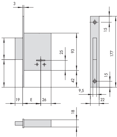
SERIE 57220 E = 40 - 45 - 50 - 60
