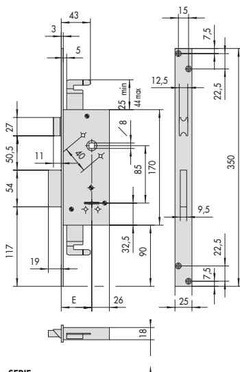
SERIE 57215 E = 45 - 50 - 60
