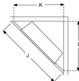
Dimensiones de la esquina empotrada
