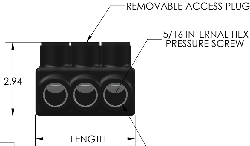
IPL500-3 SHOWN
