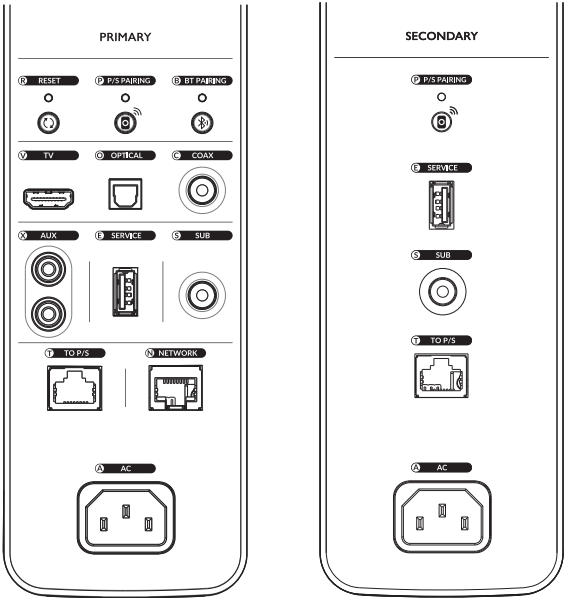
图所示, 控制和连接器位于两个音箱的后背板上。
