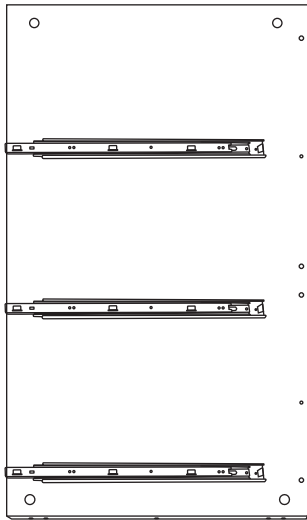
A-2. Left Side Panel A-2. Panneau latéral gauche
