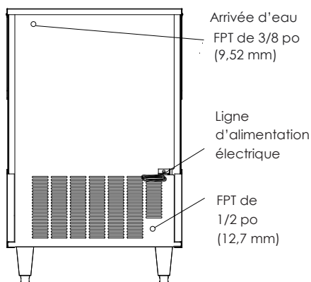
VUE DE DOS
