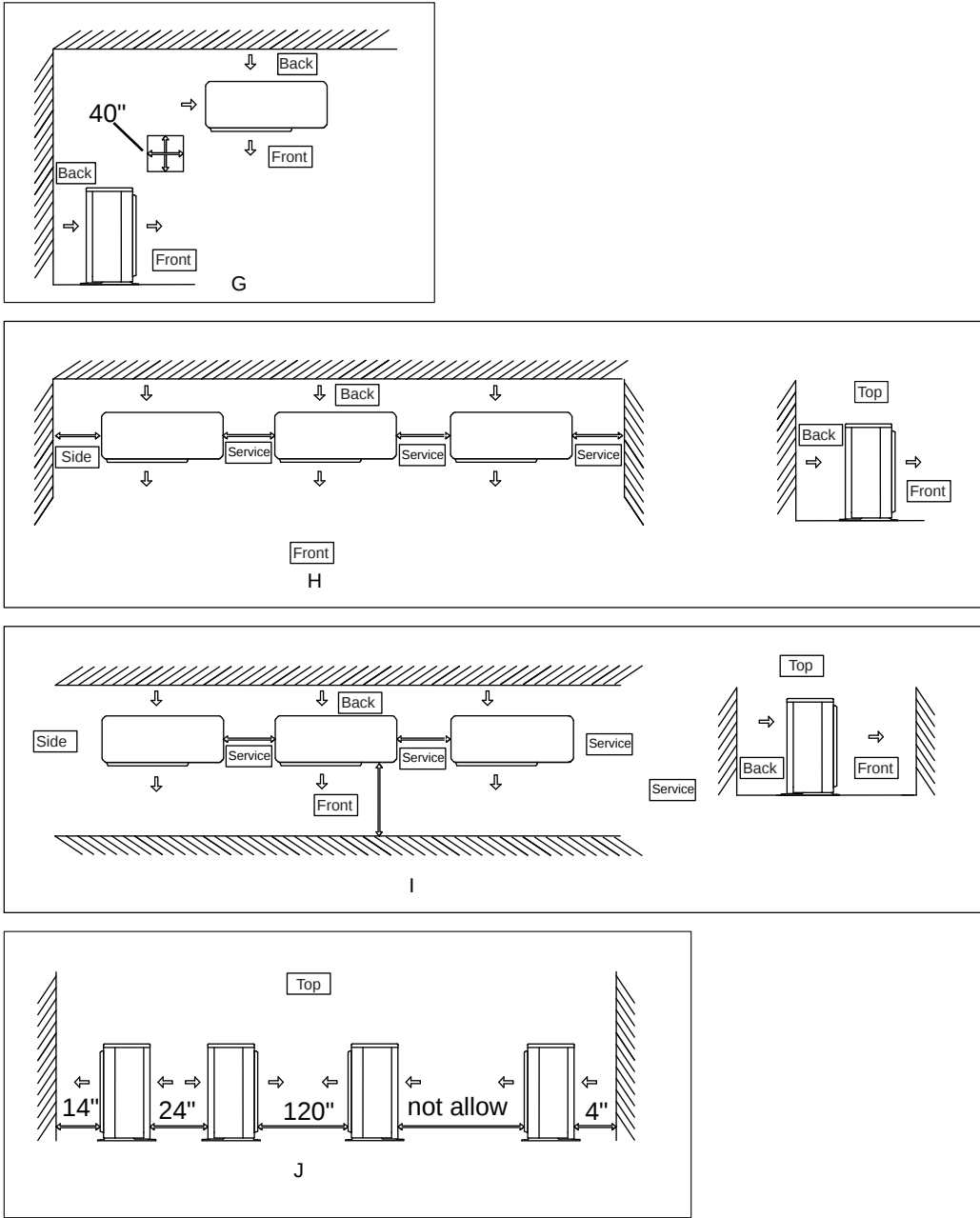
Figure 3. Configurations de dégagement pour plusieurs unités
