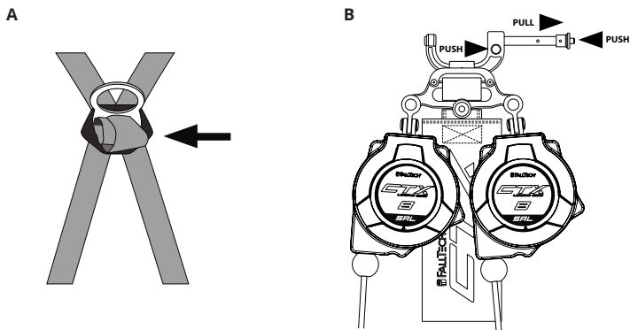
Figure 5 - Installation du bord d'attaque SRL-P de classe 2 CT-X Cable
