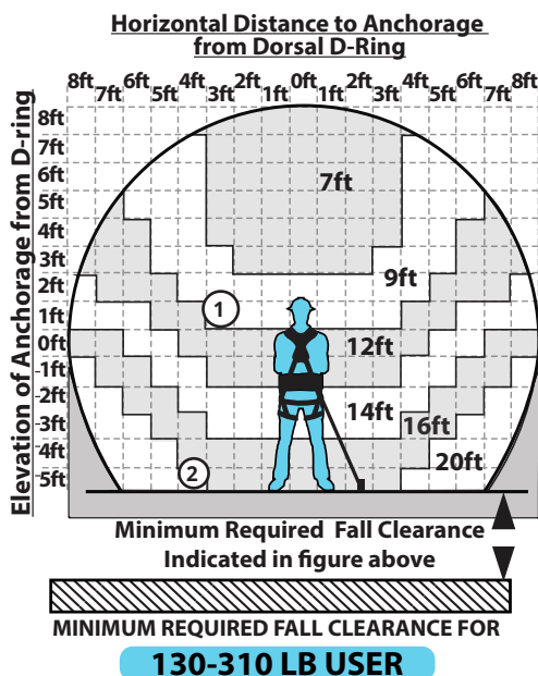
Figure 11 - Dégagement de chute minimum requis pour le CT-X pour les utilisateurs de 59 à 141 k (130 à 310 lb)
