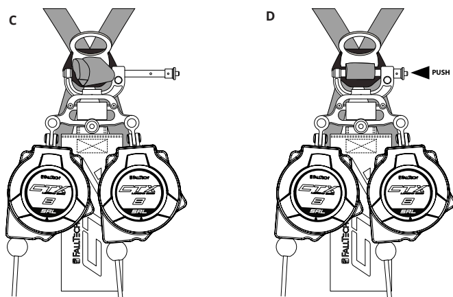
Figure 5 - Installation du bord d'attaque SRL-P de classe 2 CT-X Cable
