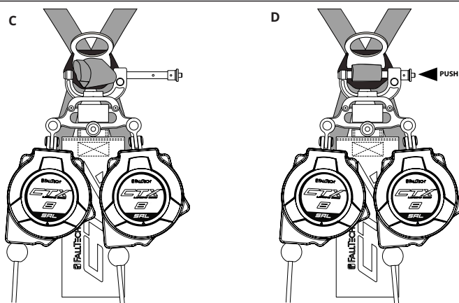
Figura 5 - Instalación de CT-X Cable Class 2 Leading Edge SRL-P
