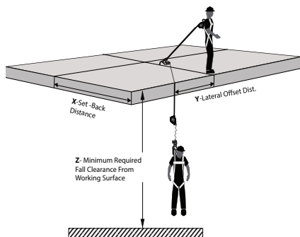
Figura 11 - Distancia despejada de caída mínima requerida de CT-X para usuarios de 130 a 310 libras (59 a 141 kg)
