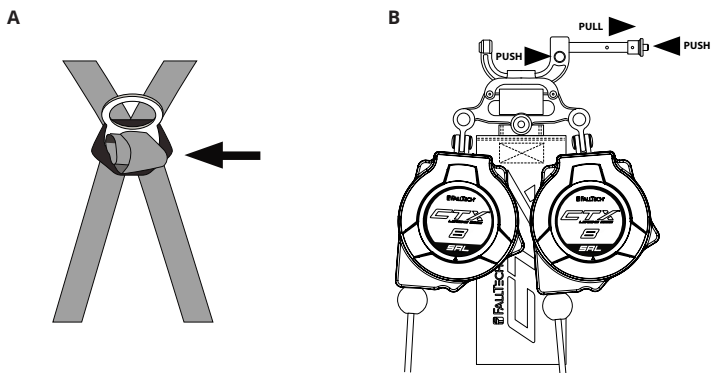
Figura 5 - Instalación de CT-X Cable Class 2 Leading Edge SRL-P
