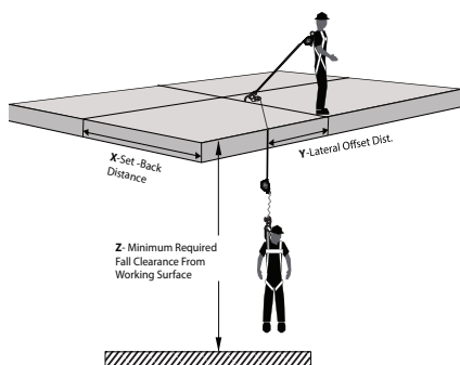
Figure 11 - Dégagement de chute minimum requis pour le CT-X pour les utilisateurs de 59 à 141 k (130 à 310 lb)
