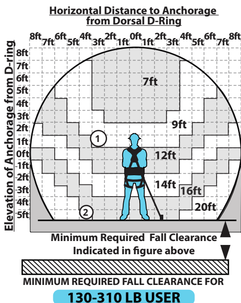
Figura 11 - Distancia despejada de caída mínima requerida de CT-X para usuarios de 130 a 310 libras (59 a 141 kg)
