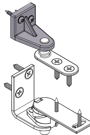
A4M00642 | SALOON DOOR HINGE KIT
