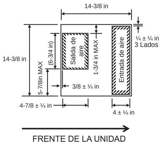
Modelos de Altura Estándar (GRCS/GRHS) VISTA DE ARRIBA HACIA ABAJO
