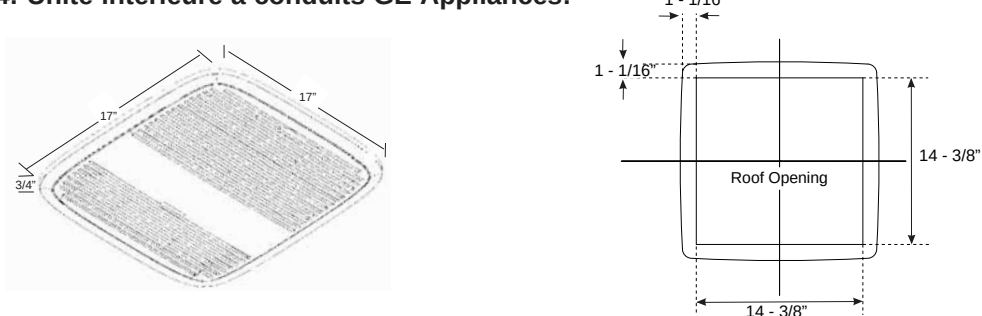
Illustration 4: Unité intérieure à conduits GE Appliances:
