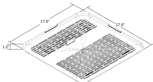
Figura 5: Unidad Interior CON Conducto de GE Profile
