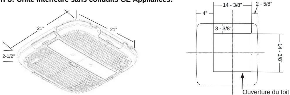
Illustration 3: Unité intérieure sans conduits GE Appliances:
