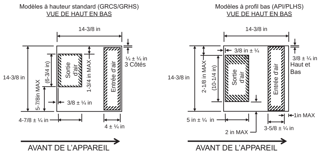
Illustration 6: Directives pour le montage de haut en bas:
