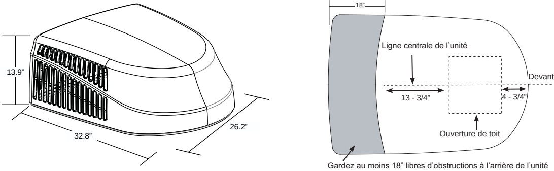
Illustration 1: Unité de toit de hauteur standard (GRCS/GRHS):
