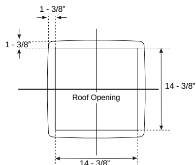
Figura 5: Unidad Interior CON Conducto de GE Profile
