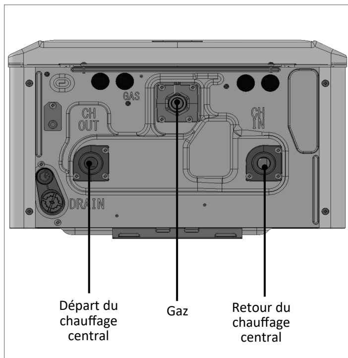
Figure 2: Vue de dessous
