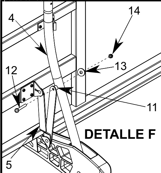
BISAGRA EN LA POSICIÓN CORRECTA
