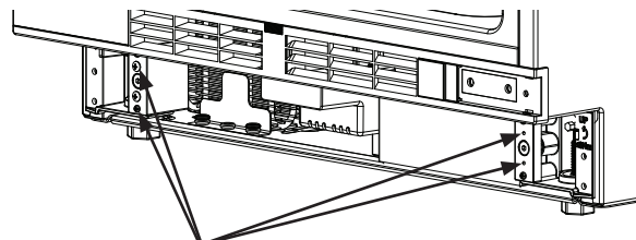
Dévisser 4 vis
