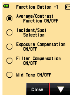
Bildschirm „Function Button -1“ (Funktionstaste -1) Seite 1
