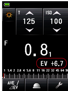
Bildschirm „Measuring“ (Messen) Zusätzliche Daten für EV-Wert
