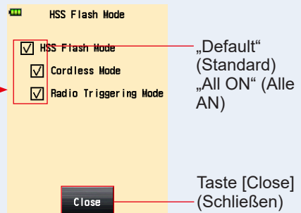
Bildschirm „HSS Flash Mode“ (HSS-Blitzmodus)
