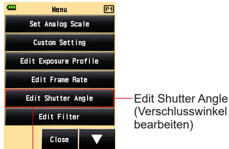
Bildschirm „Menu“ (Menü), Seite 1
