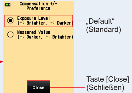
Bildschirm „Compensation +/- Preference“ (Ausgleich +/-Einstellung)
