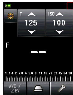
Bildschirm „Measuring“ (Messen) (Entsperren)
