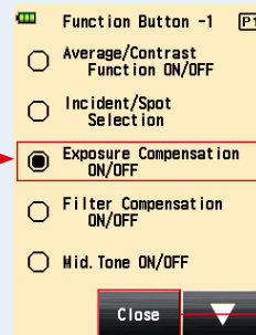
Bildschirm „Function Button -1“ (Funktionstaste -1) Seite 1
