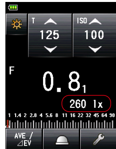
Bildschirm „Measuring“ (Messen) Zusätzliche Daten für Beleuchtungsstärke/-dichte
