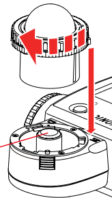
Verriegelungshebel Lichtmesshalbkugel ②①
