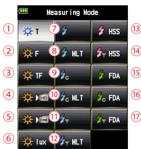
Bildschirm „Measuring Mode“ (Messmodus)
