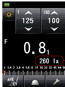
Bildschirm „Measuring“ (Messen) Zusätzliche Daten
