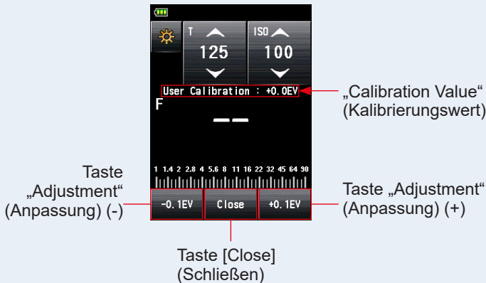
Bildschirm „User Calibration“ (Anwender-Kalibrierung)
