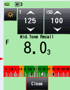
Bildschirm „Mid. Tone Recall“ (Mittelton abrufen)
