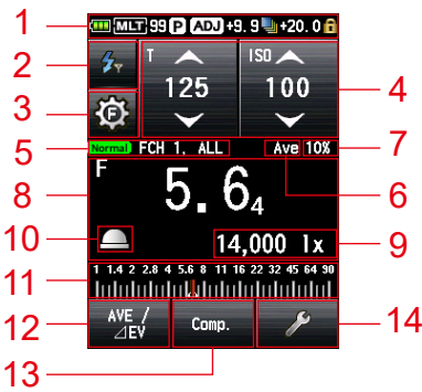
Bildschirm „Measuring“ (Messen) (Beispiel im „Radio Triggering Mode“ (Funkauslösungsmodus))
