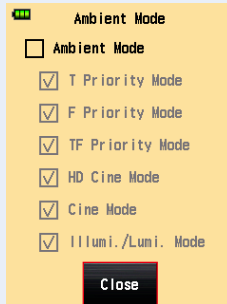
Bildschirm „Measuring Mode“ (Messmodus) Alle „OFF“ (Aus) in „Ambient Mode“ (Umgebungsmodus)
