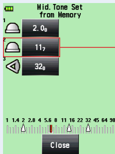
Bildschirm „Mid. Tone Set from Memory“ (Aus dem Speicher eingestellter Mittelton)
