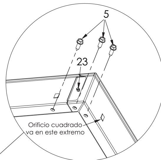
Detalle F
