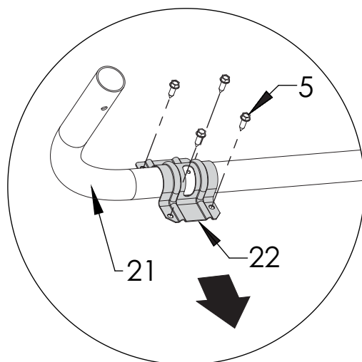
Detalle A
