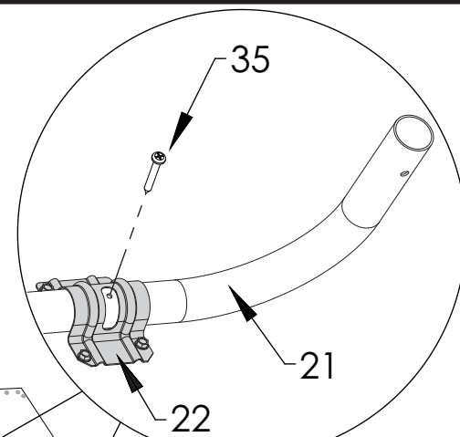
Detalle B
