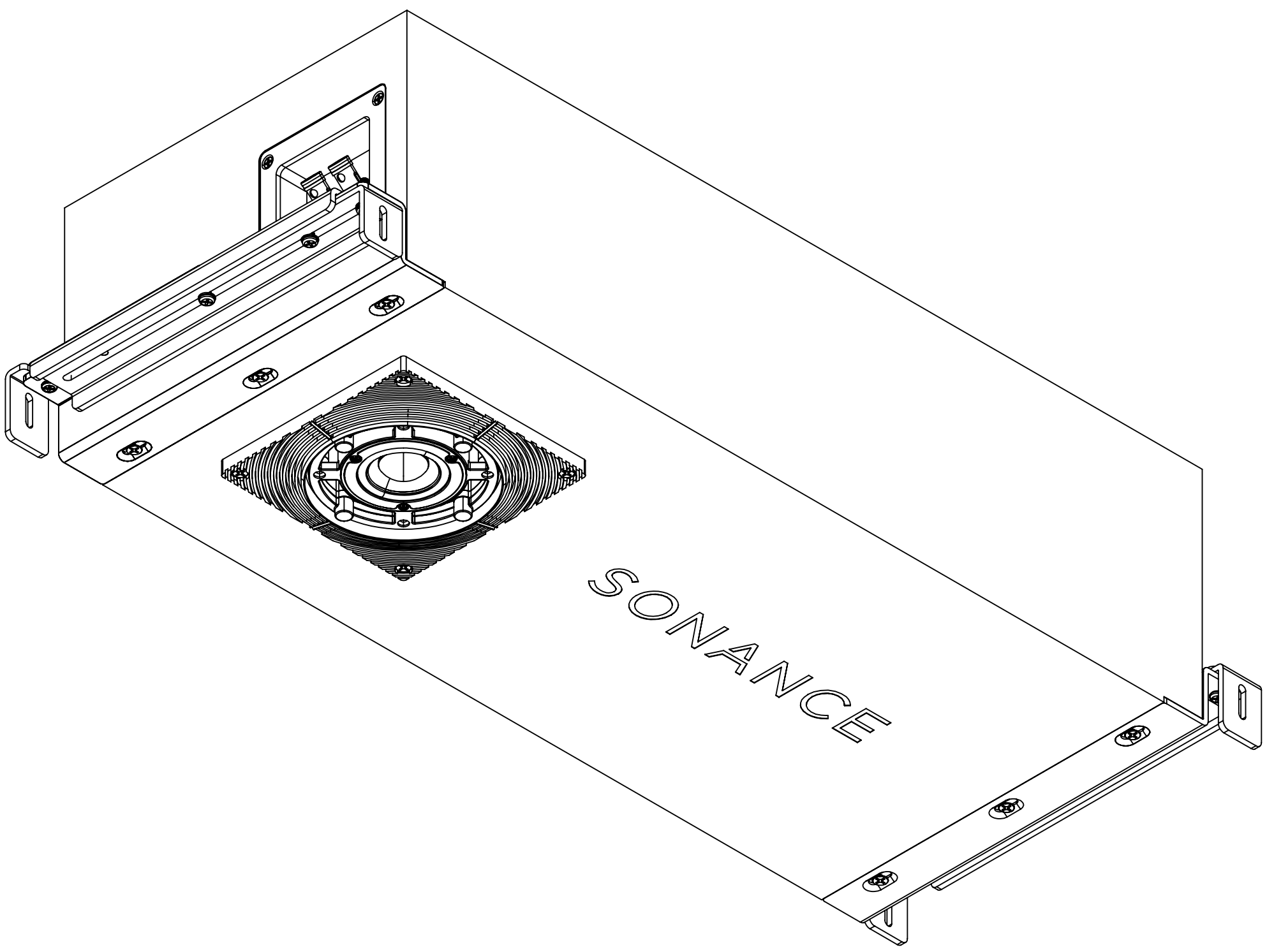
TRIMLESS GRILLE
