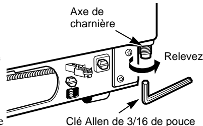
Clé Allen de 3/16 de pouce
