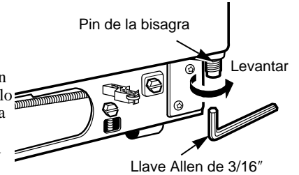
Llave Allen de 3/16"
