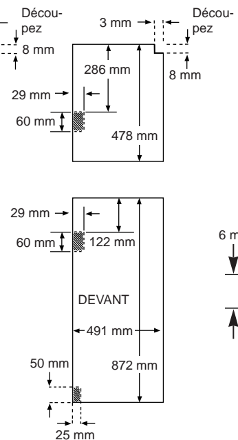
Exemple de fraisage
