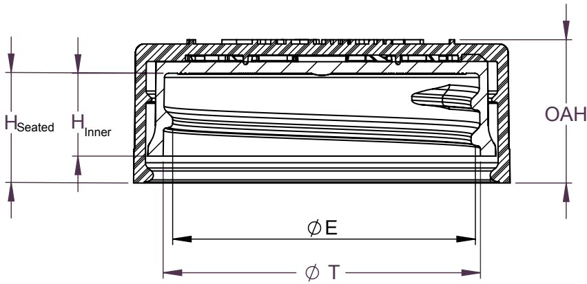
SECTION A-A SCALE 3 : 2
