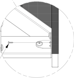
128 (x10) TORNILLO - 5/8
