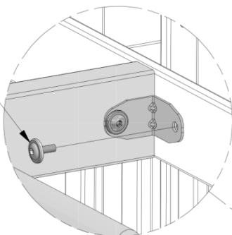
222 (x2) PERNO - 3/4"
