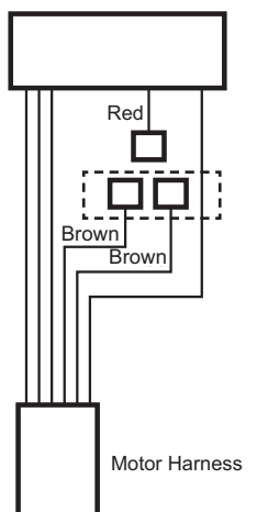
Schéma du câblage installé en usine
