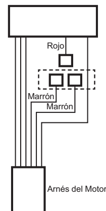
Configuración del Cableado Instalado de Fábrica
