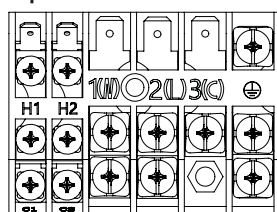
Borne de connexion de l'unité extérieure pour les modèles 115 V
