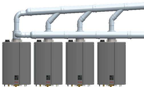
Figure 47: Exemple: Circuit commun d'évacuation Rinnai
