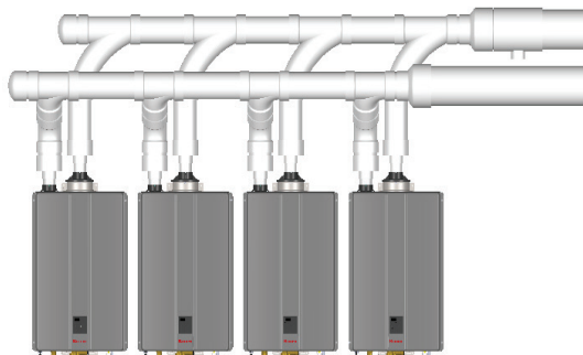
Figure 48: Exemple: Circuit commun d'évacuation PVC/CPVC Série 40
