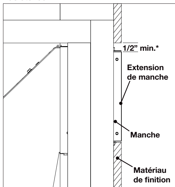
Pas étendu
