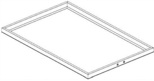
G01 ASSEMBLAGE DE PLATEAU À GRILLE -A4M02144 (x1) 1 1/4"x21 13/16"x33 1/16" (31.80x554x839)
