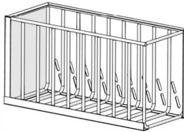
F01 BOÎTE À FEU - A4M02772 (x1) 11 11/16"x9 1/8"x22 1/2" (298x232x572)
