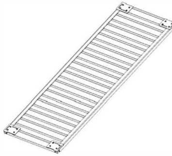
B02 ASSEMBLAGE DE LA GRILLE INFÉRIEURE - A4M02767 (x1) 1 5/8"x24 1/16"x74 3/4" (40.5x611.5x1898)
