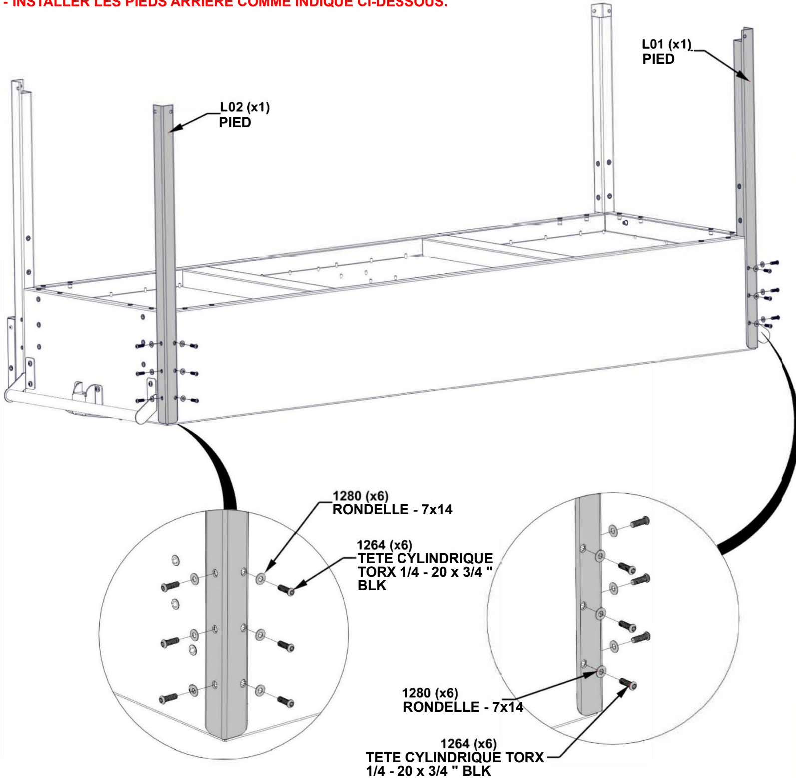
L01 PIED -A4M02912 (x1) 1 1/2"x1 1/2"x31 13/16" (38x38x808)
