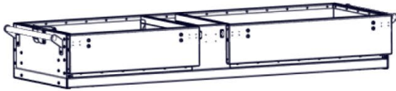
C01 ASSEMBLAGE DE BAC À CHARBON - A4M02768 (x1) 11 1/2"x25 9/16"x74 1/2" (292x650x1893)
