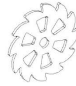
S02 PIGNON-A4M02147 (x1) 3/16"x4 11/16"x4 11/16" (4x119x119)
