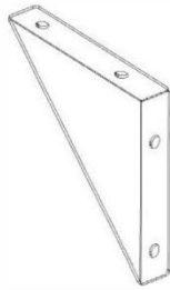
B01 ATTELLE DE PIED -A4M02910 (x8) 1"x5 3/4"x5 3/4" (26x146x146)
