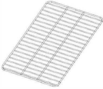
R01 GRILLE À ASADO SUPÉRIEURE - A4M02785 (x1) 5/16"x18 3/8"x26 5/16" (8x466x668)
