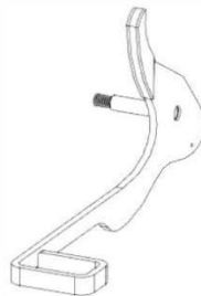
H02 ASSEMBLAGE DE POIGNÉE DE PIGNON - A4M02760 (x1) 3 5/8"x4 1/2"x9 5/16" (92x115x236)
