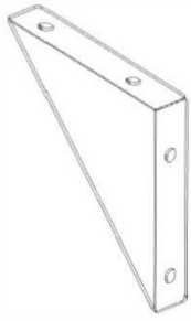
B01 ATTELLE DE PIED - A4M02910 (x8) 1"x5 3/4"x5 3/4" (26x146x146)
