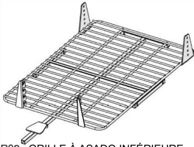
R02 GRILLE À ASADO INFÉRIEURE - A4M02786 (x1) 4 1/4"x18 1/2"x34" (108x470x864)
