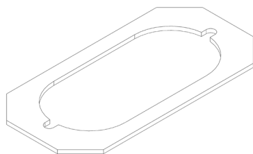
FIGURE 3 - SUPPORT POUR LE PURGEUR INTERNE
