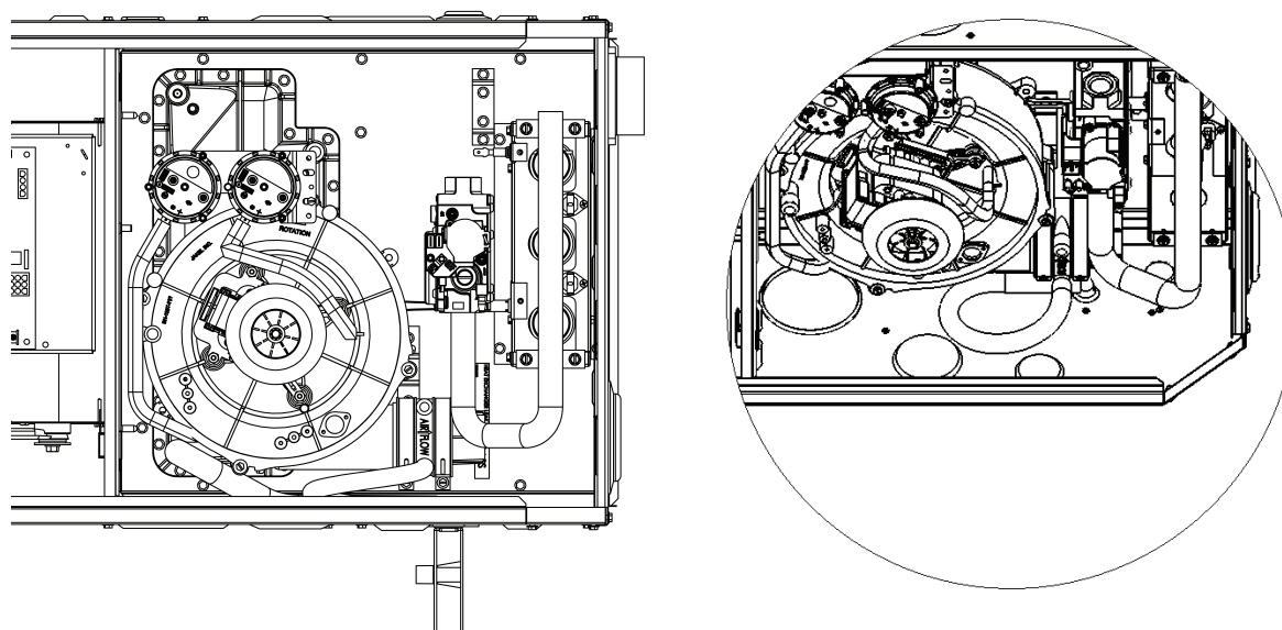
FIGURE 18 - ÉVACUATION HORIZONTALE À DROITE ET OPTION DE DRAINAGE CONTINU
