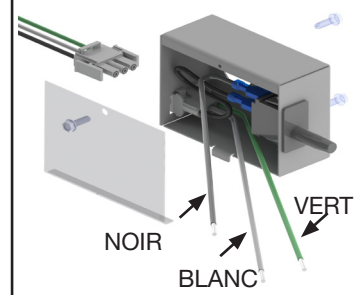
FIGURE 31 - BRANCHEMENTS ÉLECTRIQUES/CONNECTEUR MOLEX
