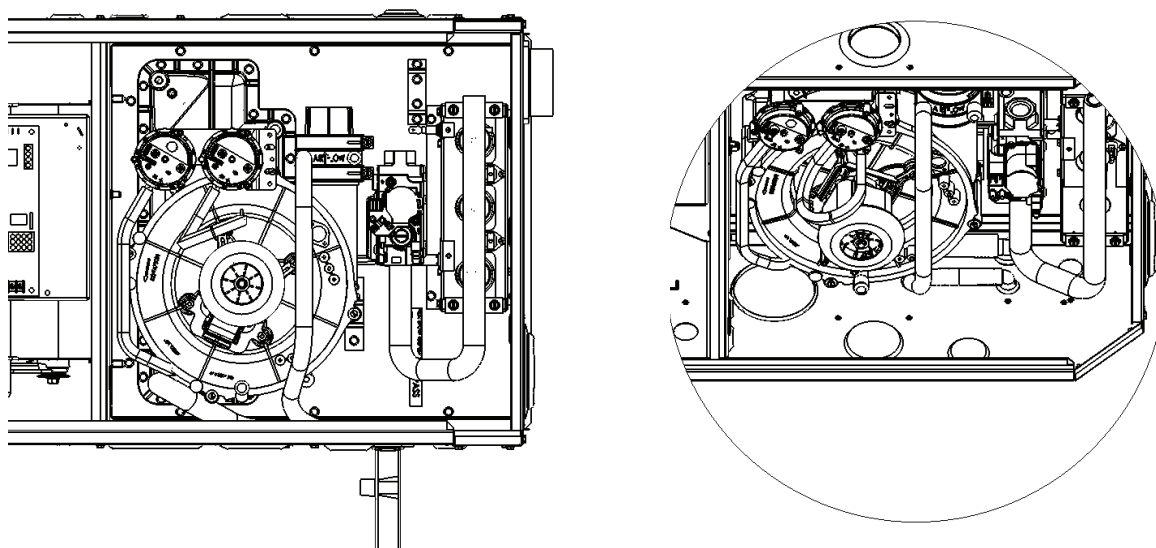
FIGURE 18 - ÉVACUATION HORIZONTALE À DROITE ET OPTION DE DRAINAGE
