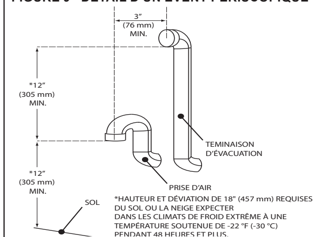
FIGURE 9 - DÉTAIL D'UN ÉVÉNEMENT PÉRISCOPEIQUE
