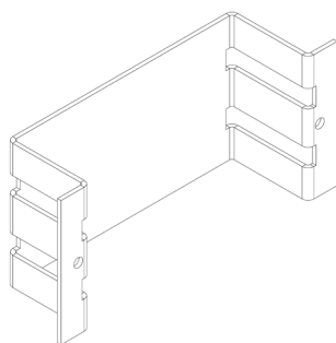
FIGURE 3 - SUPPORT POUR LE PURGEUR INTERNE
