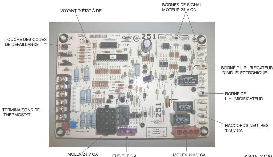
FIGURE 32 - CONTRÔLE D'ALLUMAGE DE FOURNAIE INTÉGRÉ - X13
