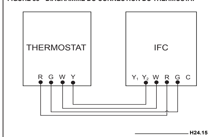
FIGURE 33 - DIAGRAMME DU CONNEXION DU THERMOSTAT
