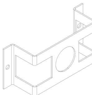
FIGURE 2 - SUPPORT POUR LE PURGEUR EXTERNE
