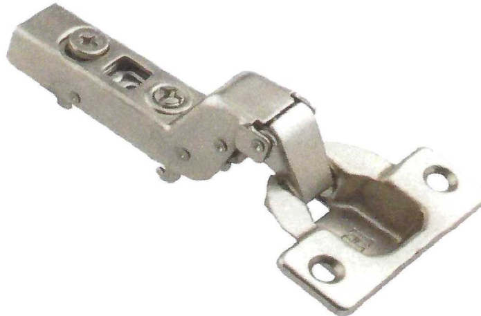
HINGE P/N 700.0537.25 shown
