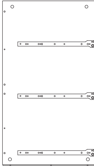
B. Right side B. Panneau latéral droit
