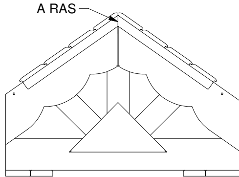
(2) RP2 - PANEL DE TEJADO SUPERIOR - W2A01514
