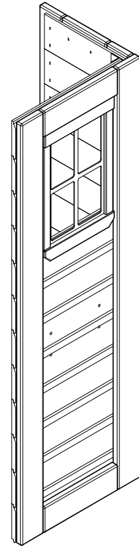
(1) WP2 - DERECHO DELANTERO ESQUINA PANEL - W2A01525
