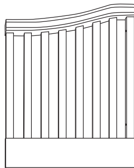
D-1. Right side panel D-1. Panneau latéral droit
