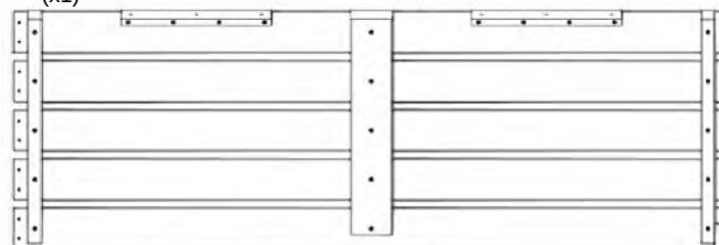
BA02 ASSEMBLAGE DE BANC GAUCHE- W2A04789 (x1) 19 1/8"x57 5/16" (50x486x1456)
