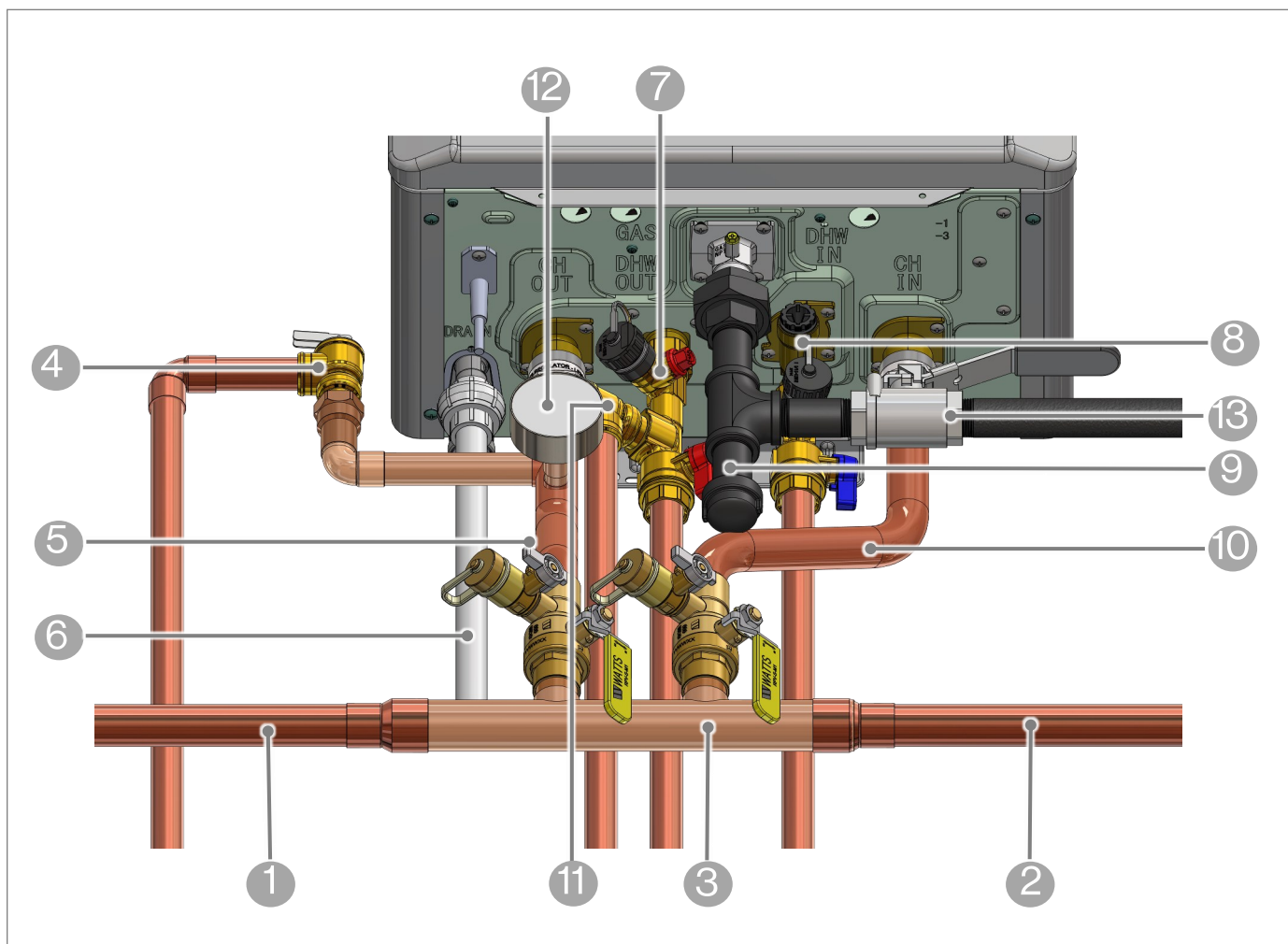
Figura 3: Vista inferior de las tuberías
