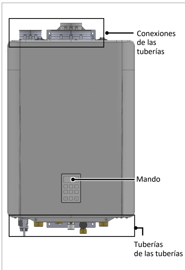
Figura 1: Vista frontal
