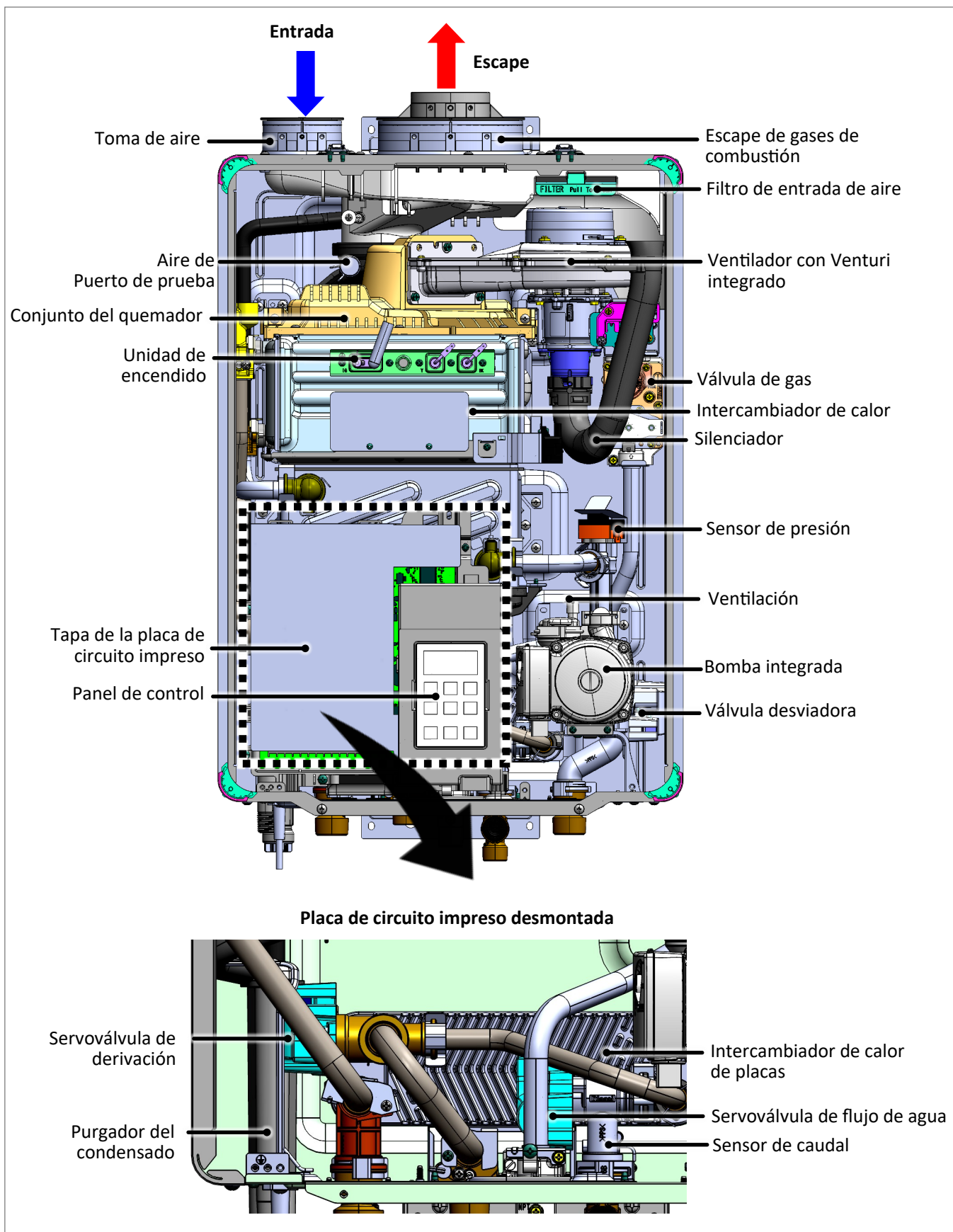
Figura 4: Componentes
