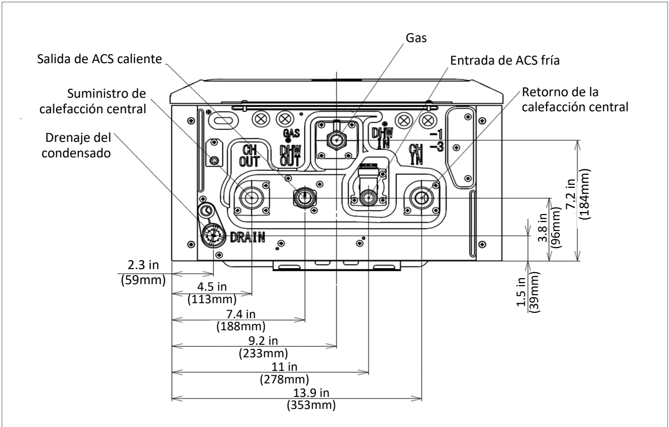
Figura 6: Conexiones de alimentación
