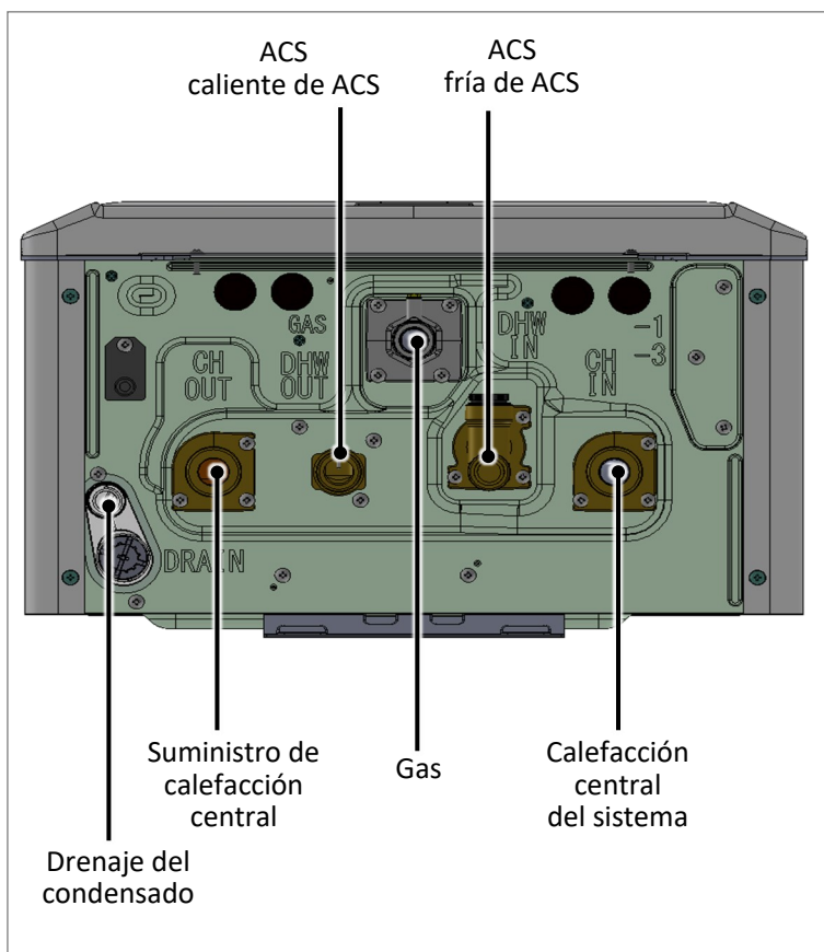
Figura 2: Vista inferior
