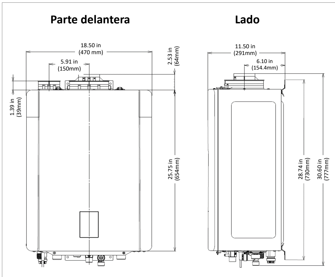
Figura 5: Dimensiones
