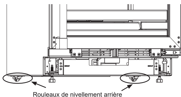
Vis de réglage du rouleau de nivellement arrière
