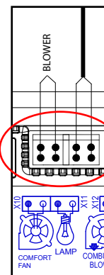
VENTILATEUR/ LAMPE BORNIER
