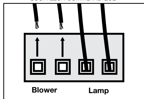
VENTILATEUR/LAMPE BORNIER (VUE DE DESSUS)
